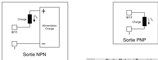
Sortie Relais / Transistor – PA 12 A/B
